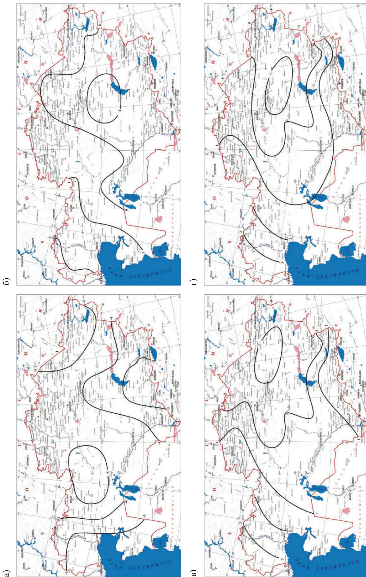
Рисунок 5. Аномалии температуры воздуха ( ^{\circ}\text{C} ) для формы циркуляции E а) зима, б) весна, в) лето, г) осень
