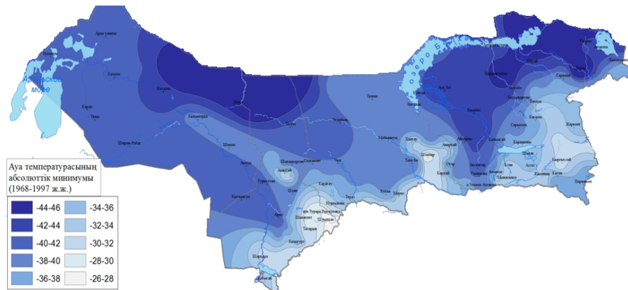
1-сурет – Оңтүстік Қазақстандағы ауа температурасының абсолюттік минимум мәндерінің таралуы (1968 – 1997 жылдар аралығы)
