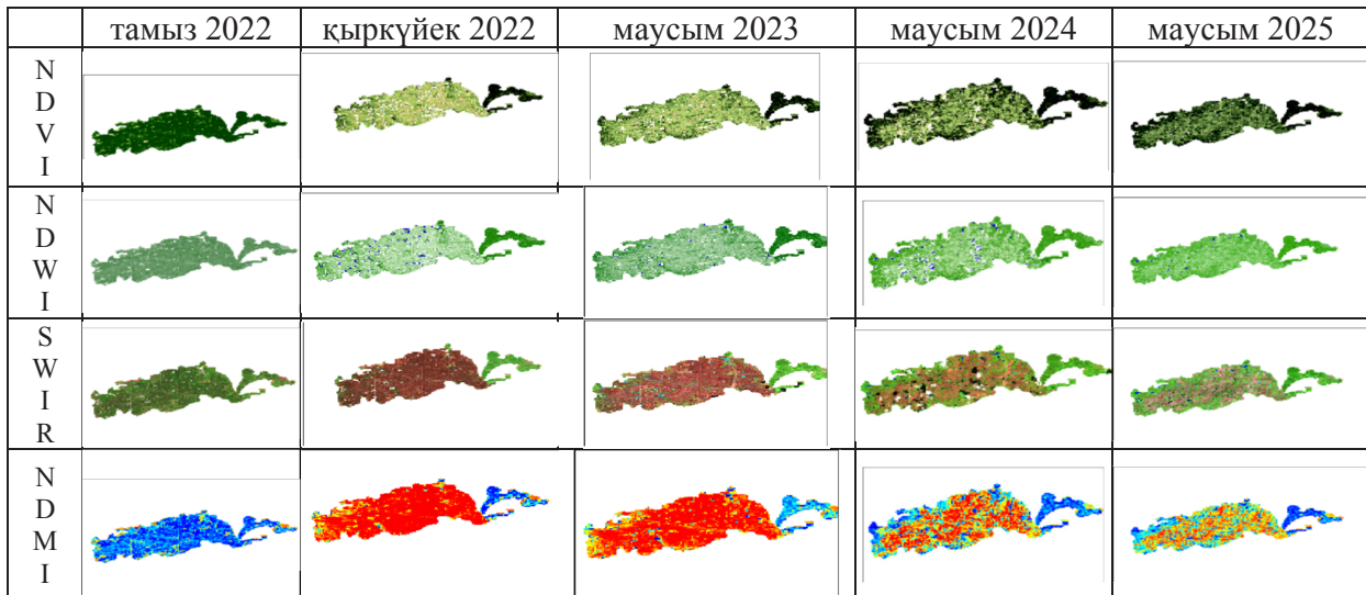
7-сурет – Sentinel-2 L2A бойынша NDVI, NDWI, SWIR, NDMI есептеу
